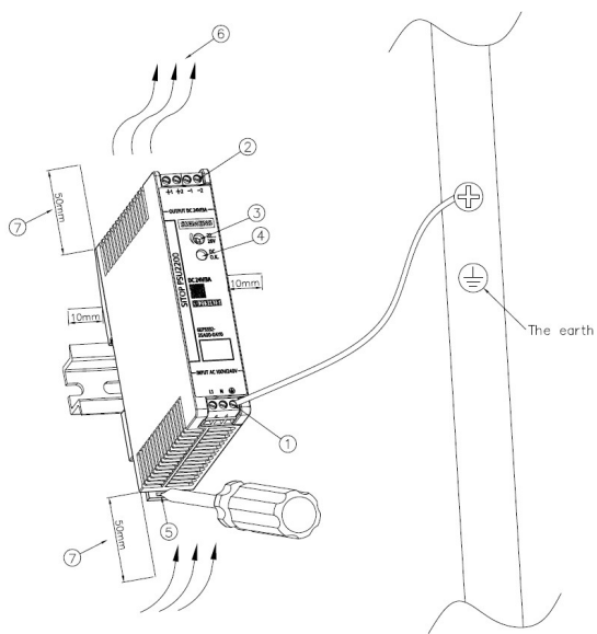
图 4: 导轨安装方式和安装空间
